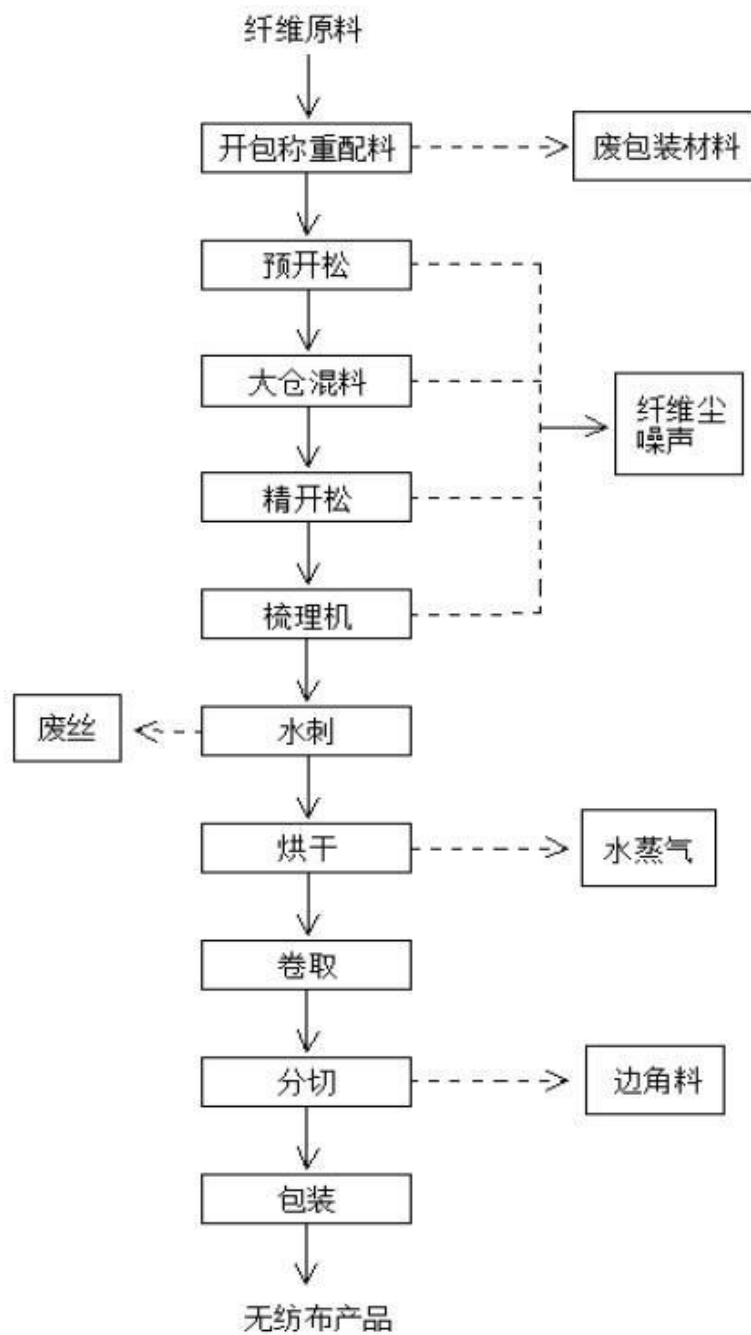
图 2-3 双梳直铺工艺流程及产物节点图
