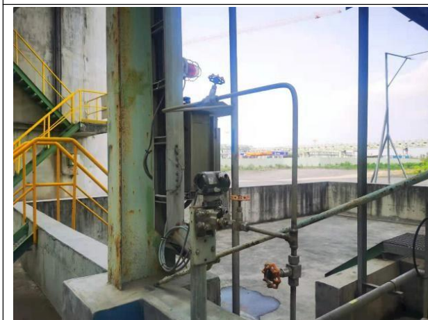
氨水泄漏检测和警报装置
