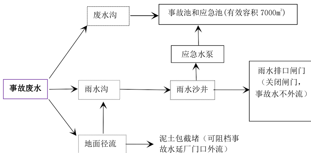
图 2-7 事故废水收集系统示意图
