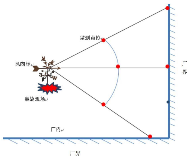
图 6-4 厂内大气应急采样点的布设示意图
