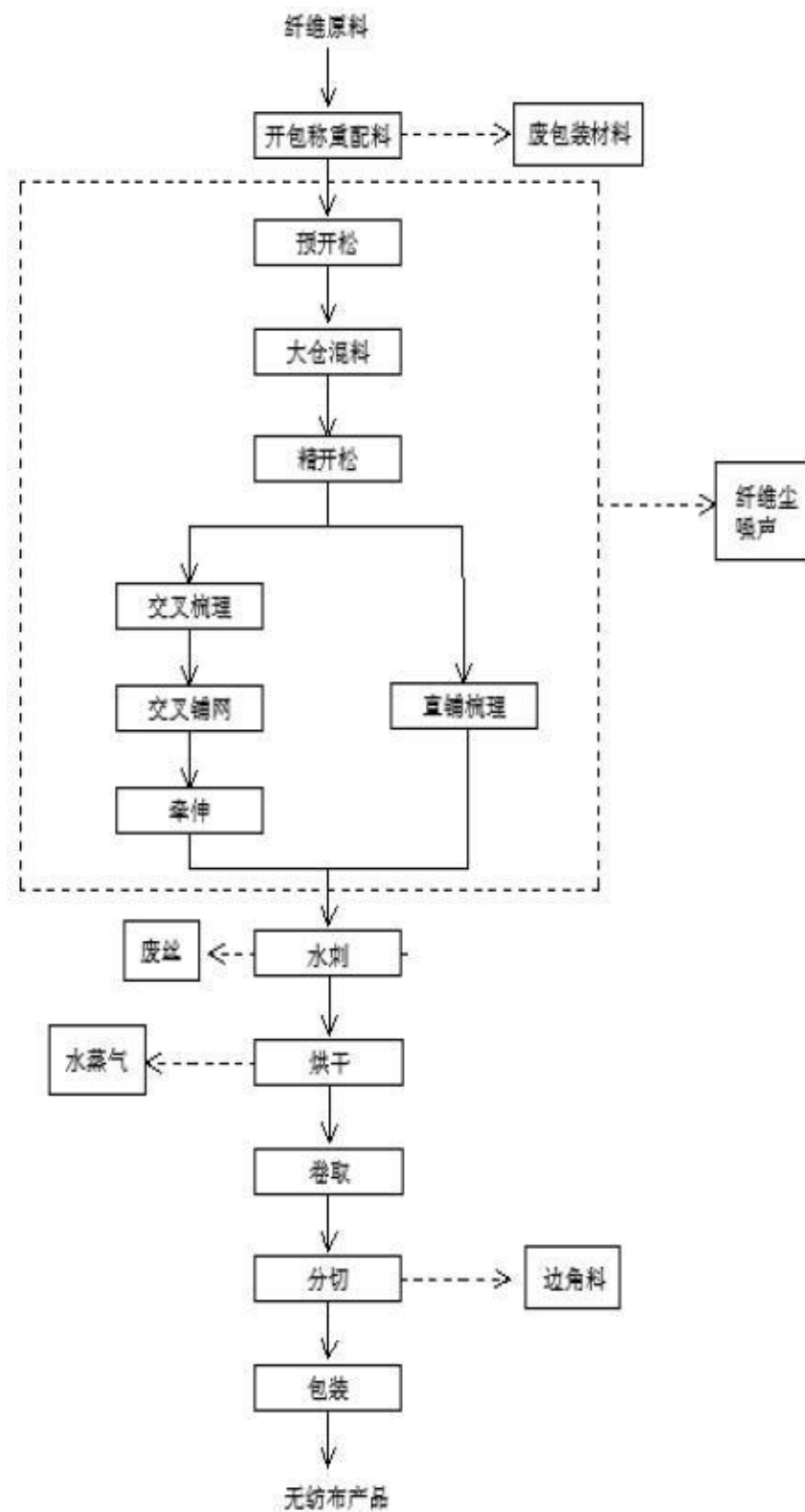
图 2-4 双梳半交铺工艺流程及产物节点图
