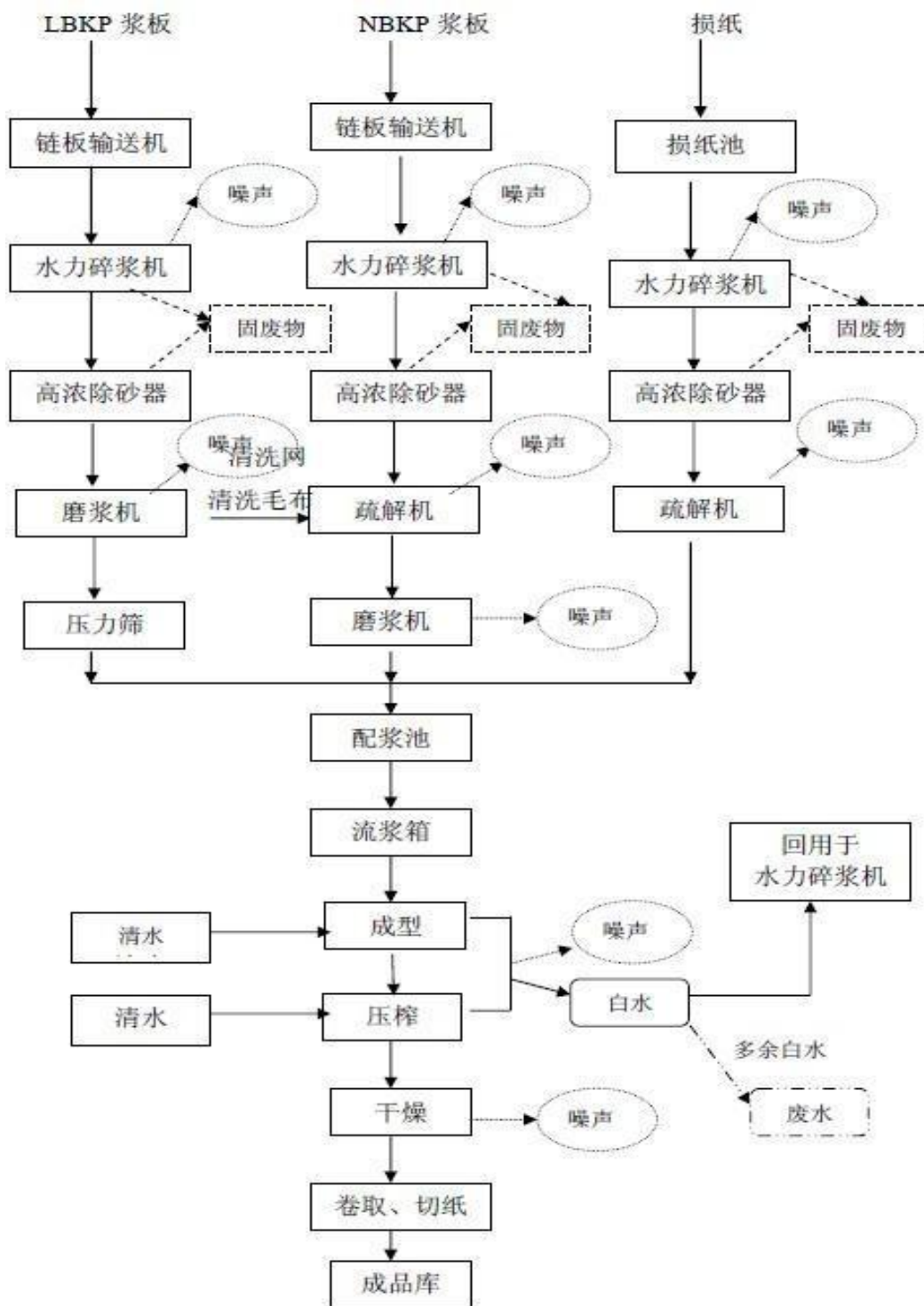
图 2-2 主要生产工艺
