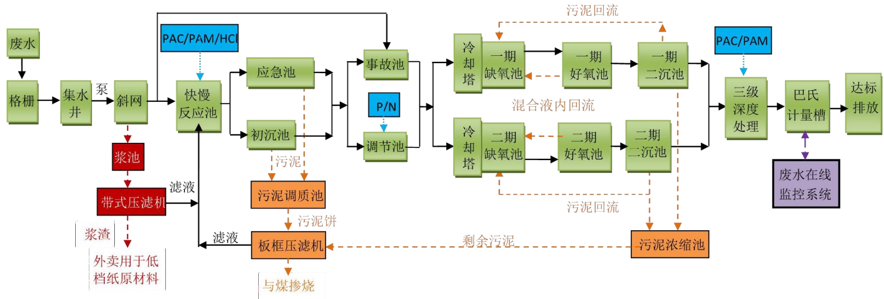
图2-5 废水处理工艺流程图
