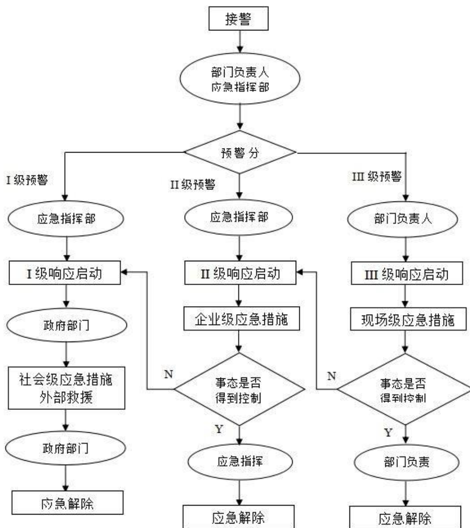
图 6-1 突发环境事件应急响应程序
