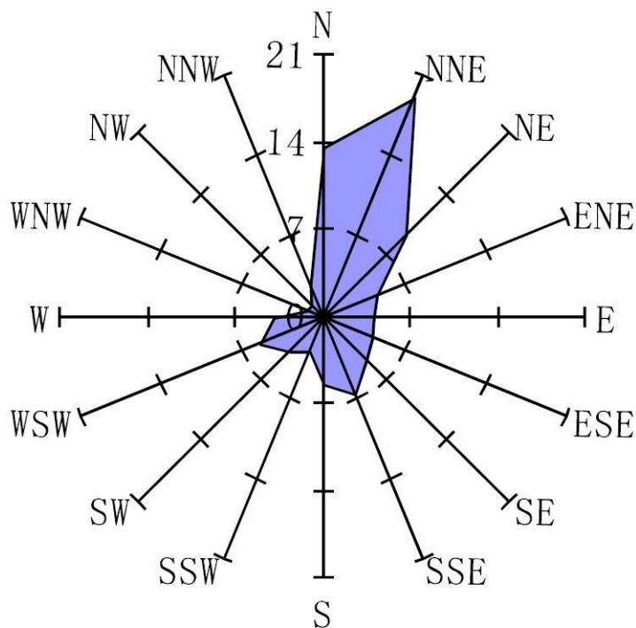
图 2-1 新会区年风向频率玫瑰图（静风频率 8.1%）
